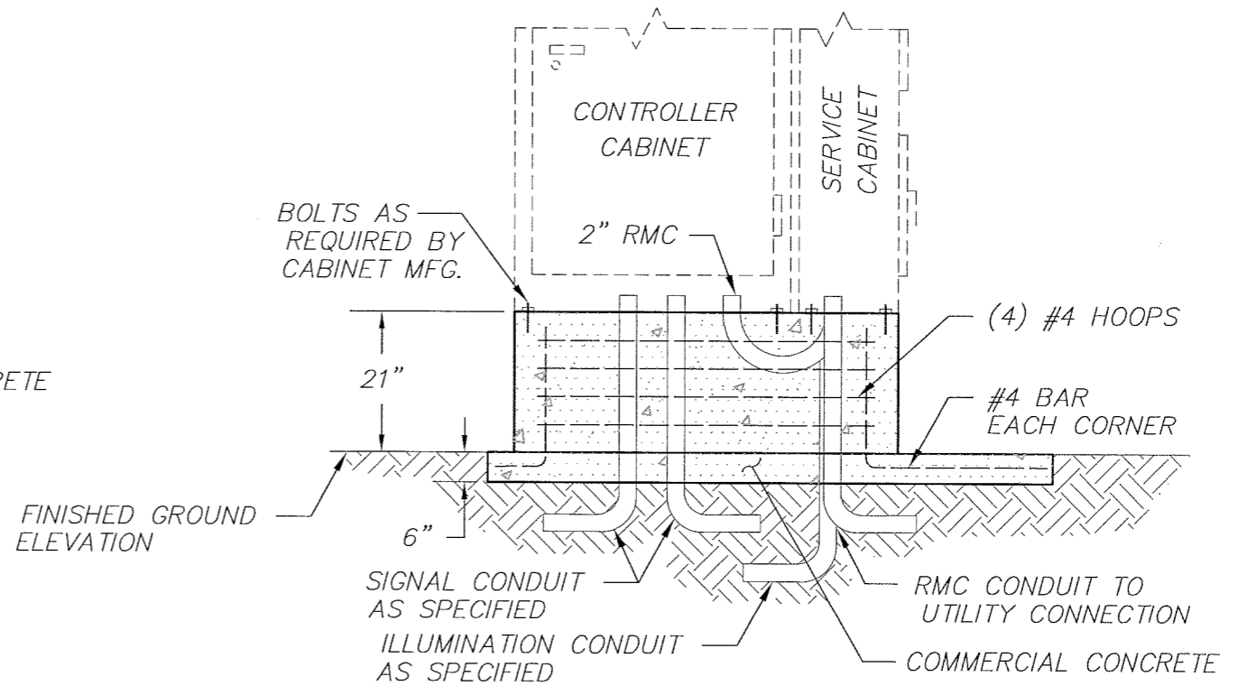
ELEVATION
